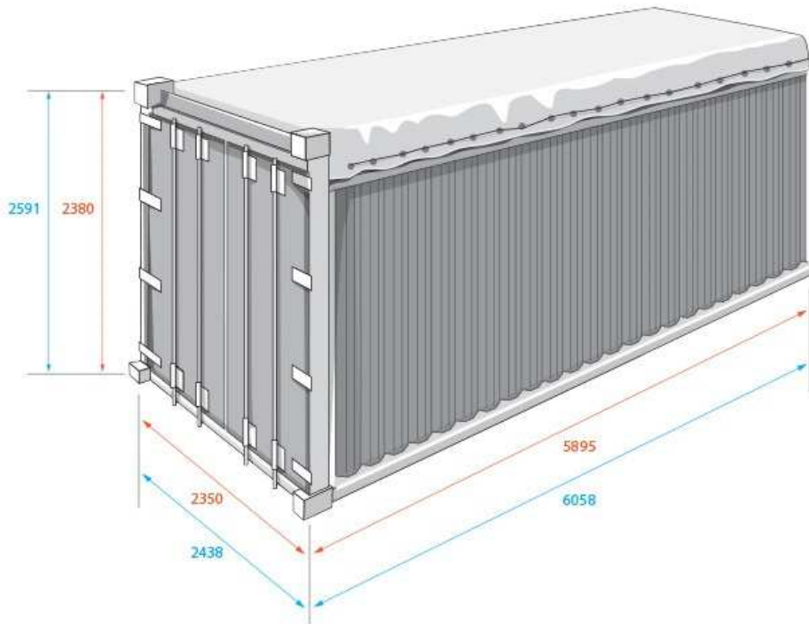
MODEL: 20' OT wymiary wewnętrzne (mm) wymiary zewnętrzne (mm)
