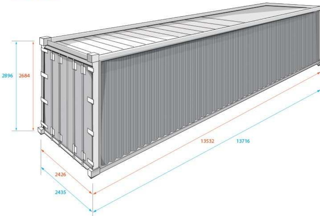
MODEL: 45' HC wymiary wewnętrzne (mm) wymiary zewnętrzne (mm)
