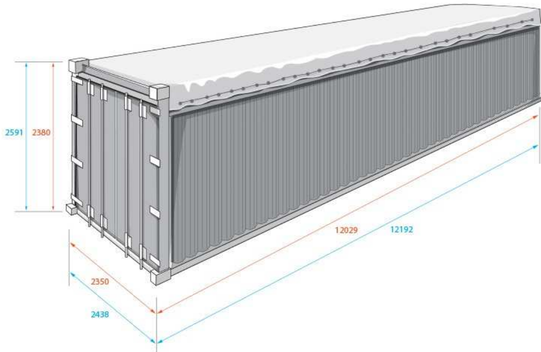
MODEL: 40' OT wymiary wewnętrzne (mm) wymiary zewnętrzne (mm)
