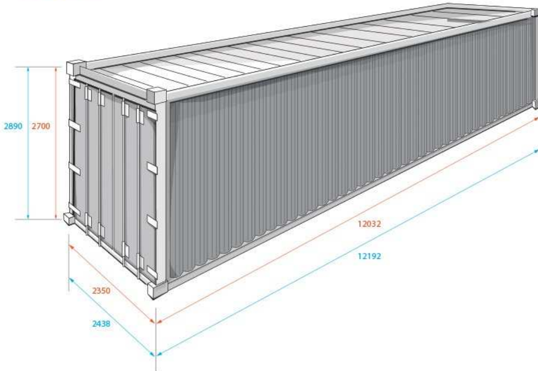
MODEL: 40' HC wymiary wewnętrzne (mm) wymiary zewnętrzne (mm)
